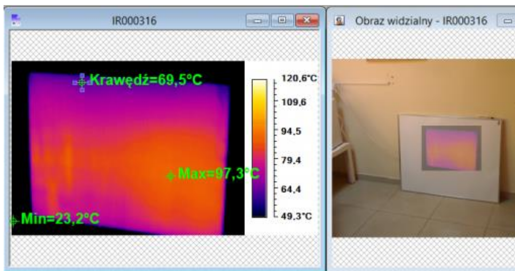
Nierówny rozkład temperatury na powierzchni grzewczej
